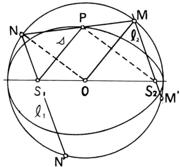
図6 卵形線 定義3
