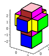
図 10 分割 (4, 3, 2)
