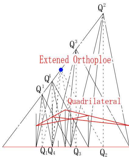
Step 2 (Chain 4)
