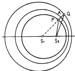
図3 卵形線 定義1
